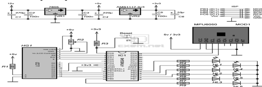
Рис 1. Схема подключения MEMS в систему с БОС
